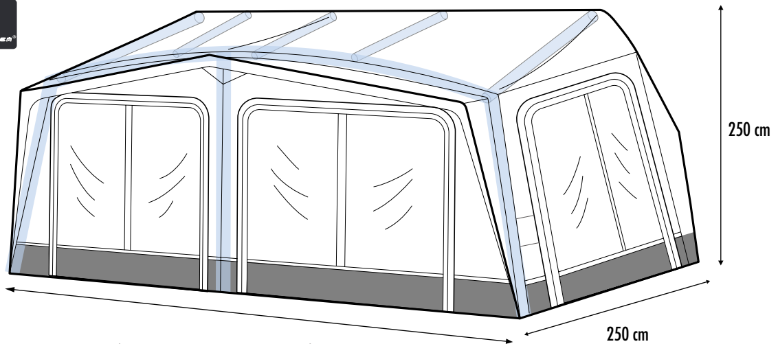
Umlaufmaß/ A-Frame-Size
